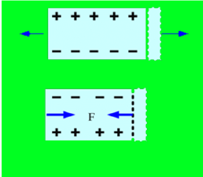
Прямой пьезоэффект
